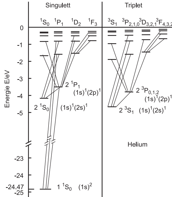
Termschema von Helium
